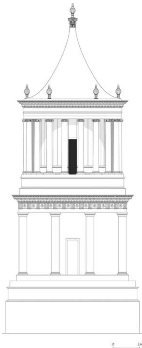
איור 2: שחזור מבנה המאוזולאון (איור: רחל צ'אצ'י)
